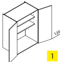
BA Buffet-Aufsatzzschrank ↔ 80/90/100/120 ↑ 120/135/150 ↘ 50
