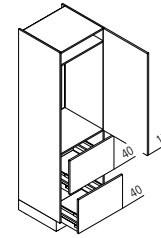
GKZ Geräteschrank für Kühlschrank / Nische 102,5 cm
