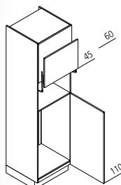
GKL Geräteschrank mit Lifttür für Mikrowelle, Kühlschrank / Nische 102,5 cm
