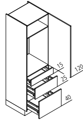
GKAK Geräteschrank für Kühlschrank / Nische 88 cm
