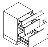
UAK Auszugsschrank
