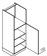
GB Geräteschrank für Backofen oder Mikrowelle
