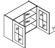
HVSP Hängeschränk mit Glastür (programmabhängig) ↔ 80/90/100/120 ↓ 60/75/90 ↙ 35
