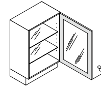
UDDDN Unterschrank mit Glastür DN ↔ 40/45/50/60 ↑ 80 ↘ 39
