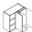
HES Hängeschränk-Ecke
