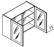
HVDN Hängeschränk mit Glastür DN ↔ 80/90/100/120 ↓ 60/75/90 ↙ 35
