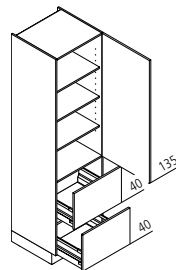
VZ Vorratsschrank
