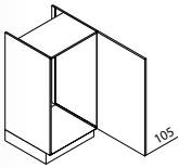
GK Geräteschrank für Kühlschrank / Nische 102,5 cm ↳ 60 ↳ 105 ↳ 60
