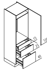
GKAK Geräteschrank für Kühlschrank / Nische 102,5 cm
