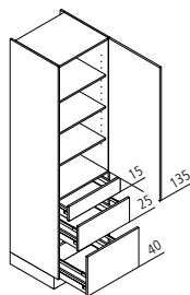
VAK Vorratsschrank
