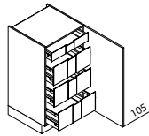
VI Vorratsschrank ↳ 40/45/50/60 ↳ 105 ↳ 60/50/35
