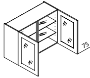
HV Hängeschränk mit Glastür (programmabhängig) ↔ 80/90/100/120 ↓ 60/75/90 ↙ 35
