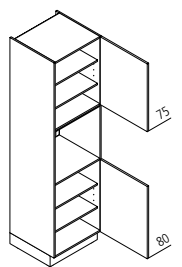
GB Geräteschrank für Backofen oder Mikrowelle
