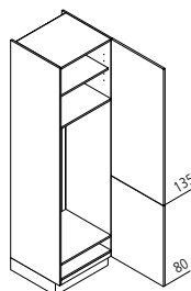
GKG Geräteschrank für Kühl- Gefrierkombination / Nische 144 cm
