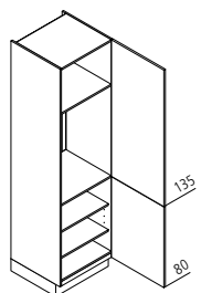
GK Geräteschrank für Kühlschrank / Nische 88 cm
