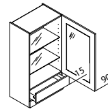
HASKV Aufsatzzschrank mit Glastür (programmabhängig) ↔ 45/50/60 ↑ 115 ↘ 35
