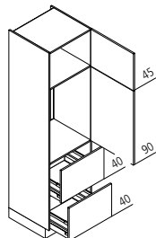
GKZ Geräteschrank für Kühlschrank / Nische 88 cm
