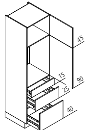
GKAK Geräteschrank für Kühlschrank / Nische 88 cm
