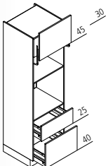
GBLAZ Geräteschrank mit Lifttür für Mikrowelle, Backofen
