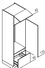
GKA Geräteschrank / Nische 102,5 cm
