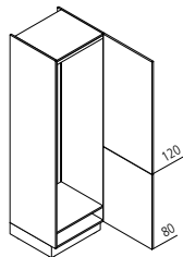
GKG Geräteschrank für Kühl- Gefrierkombination / Nische 178 cm
