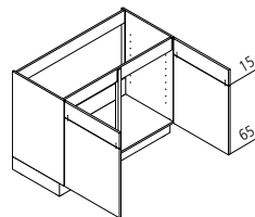
SO Spülenunterschrank
