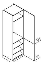
GK Geräteschrank für Kühlschrank / Nische 102,5 cm
