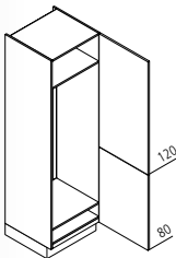
GKG Geräteschrank für Kühl- Gefrierkombination / Nische 144 cm
