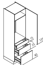
GKAK Geräteschrank für Kühlschrank / Nische 102,5 cm
