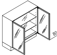
UDDDR Unterschrank mit Glastür DR ↔ 80/90/100/120 ↑ 80 ↘ 39
