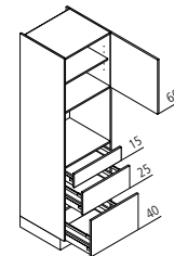
GBAK Geräteschrank für Backofen oder Mikrowelle
