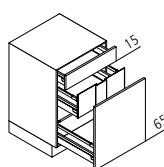
UATIA Auszugsschrank/ Topfschrank
