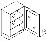
UDDV Unterschrank mit Glastür (programmabhängig) ↔ 40/45/50/60 ↑ 80 ↘ 60/39
