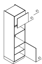
GBL Geräteschrank mit Lifttür für Mikrowelle, Backofen
