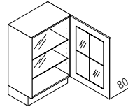
UDDVSP Unterschrank mit Glastür (programmabhängig) ↔ 40/45/50/60 ↑ 80 ↘ 60/39
