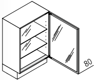
UDDDR Unterschrank mit Glastür DR ↔ 40/45/50/60 ↑ 80 ↘ 39
