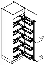
VVK Vorratsschrank
