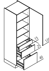
VAK Vorratsschrank
