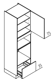
GBBA Geräteschrank für Backofen und Mikrowelle
