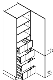
VI Vorratsschrank
