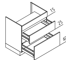
KAK Kochstellenschrank für Muldenlüfter
