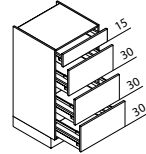
VAK Vorratsschrank ↳ 30/40/45/50/60 ↳ 105 ↳ 60/50
