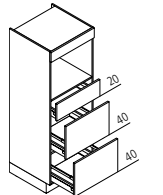
GBZ Geräteschrank für Backofen oder Mikrowelle
