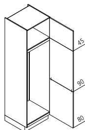
GK Geräteschrank für Kühlschrank / Nische 159 cm
