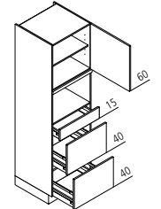
GBZ Geräteschrank für Backofen oder Mikrowelle
