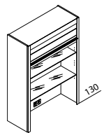
HAJGO Aufsatzzschrank mit Jalousie in Glas-Optik ↔ 60/90 ↑ 115/130/145 ↘ 35/50/60 Lieferbar in Schwarz softmatt oder Schwarz Hochglanz
