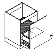
SABD Spülenunterschrank mit Abfalltrennsystem
