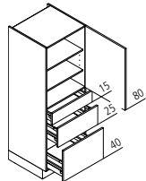
VAK Vorratsschrank
