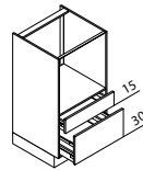
GBAS Geräteschrank für Backofen oder Mikrowelle ↳ 60 ↳ 105 ↳ 60
